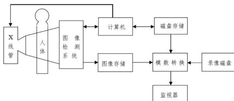
图 9-2 DSA 系统结构图
