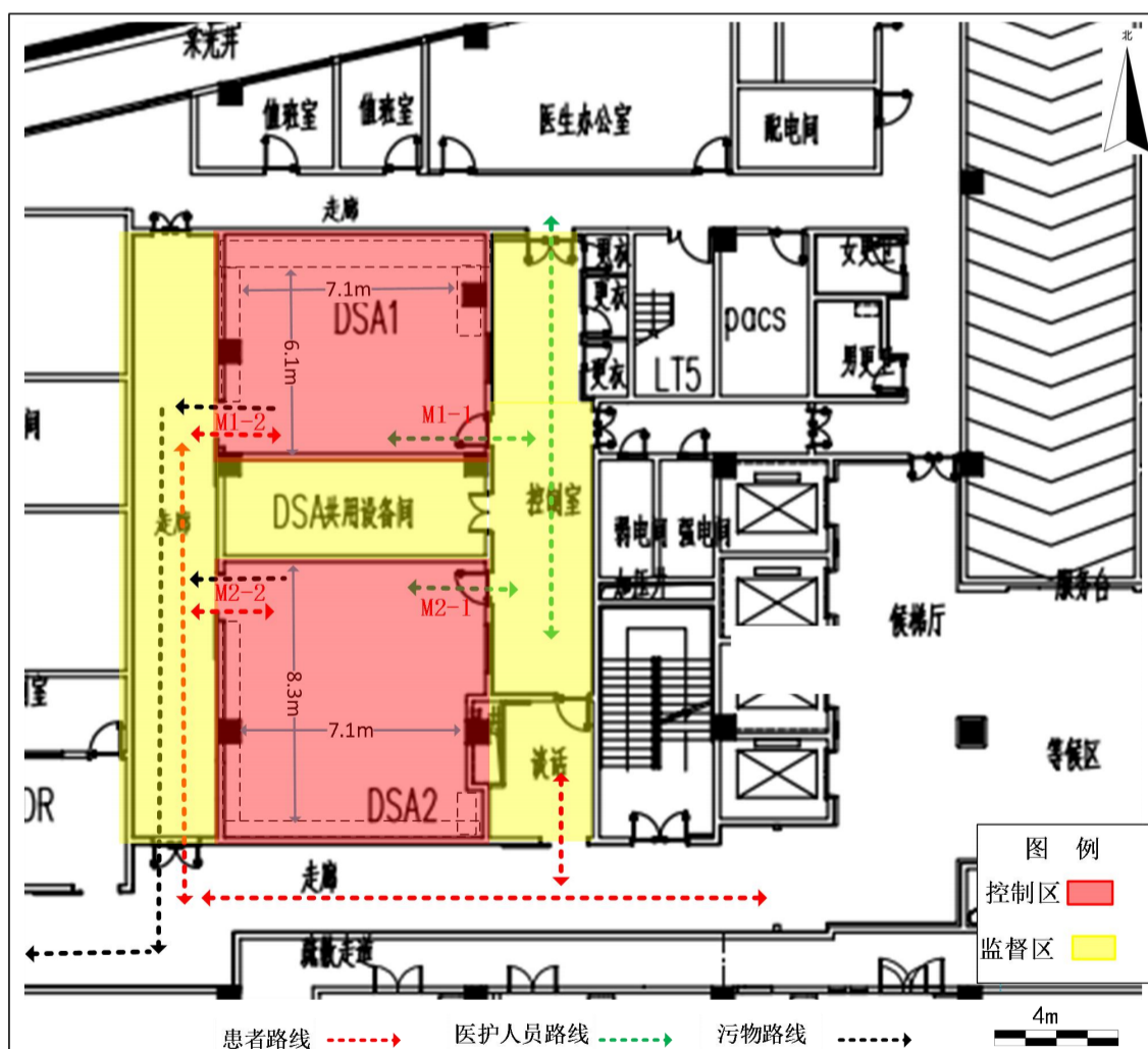
图 10-1 本项目 DSA 工作场所平面布置、分区及人流、物流路径示意图
