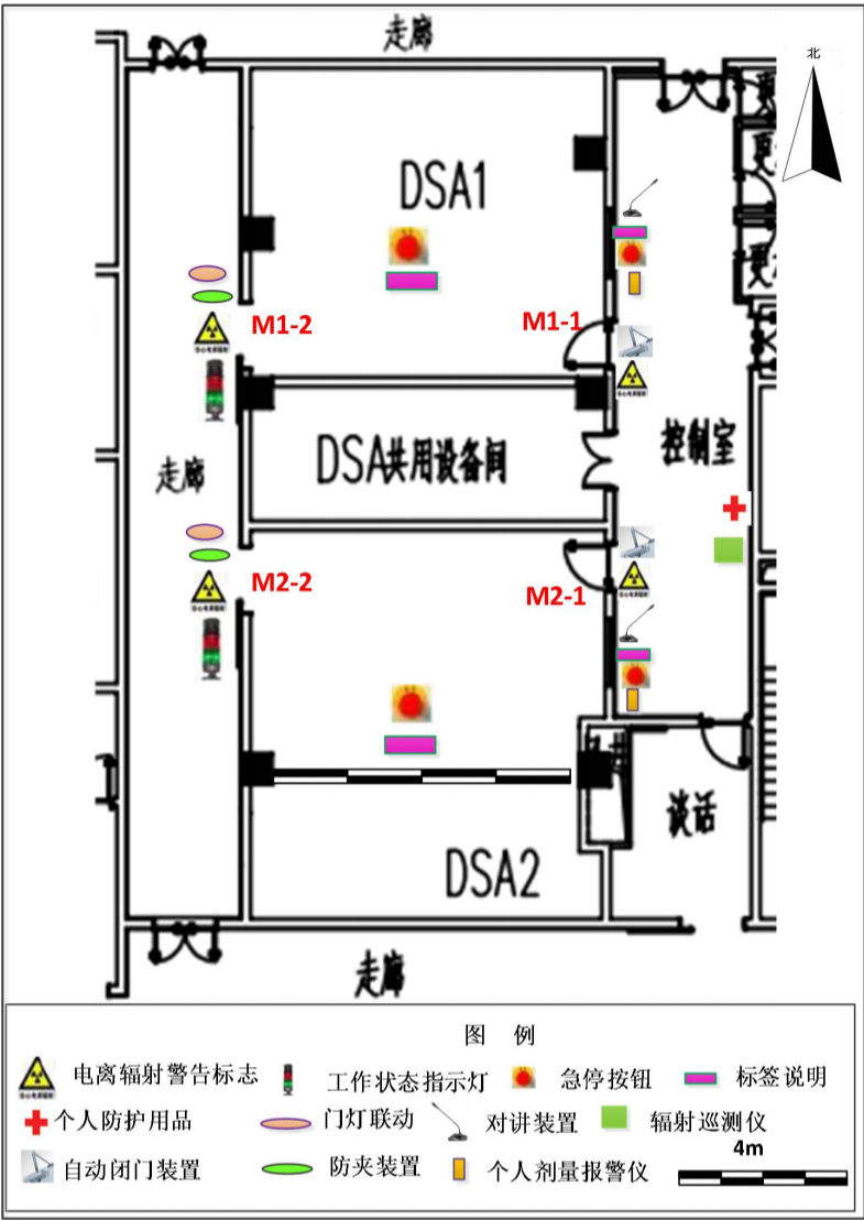
图 10-2 本项目 DSA 机房辐射安全与防护设施分布示意图
