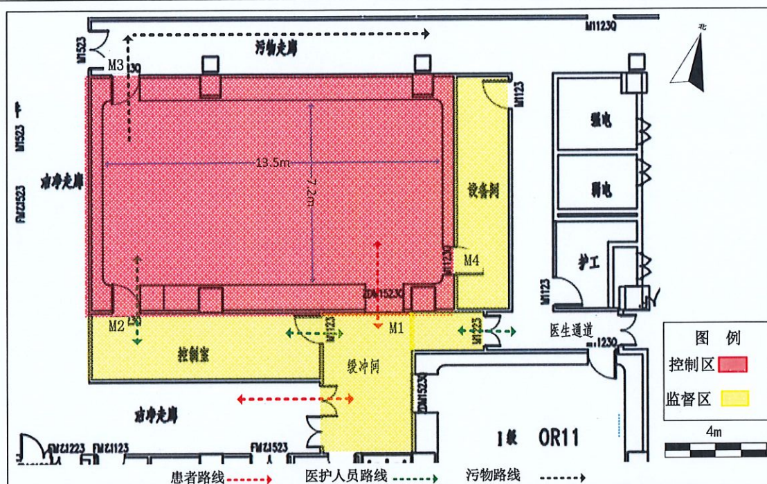
图 10-1 本项目 DSA 工作场所平面布置、分区及人流、物流路径示意图
