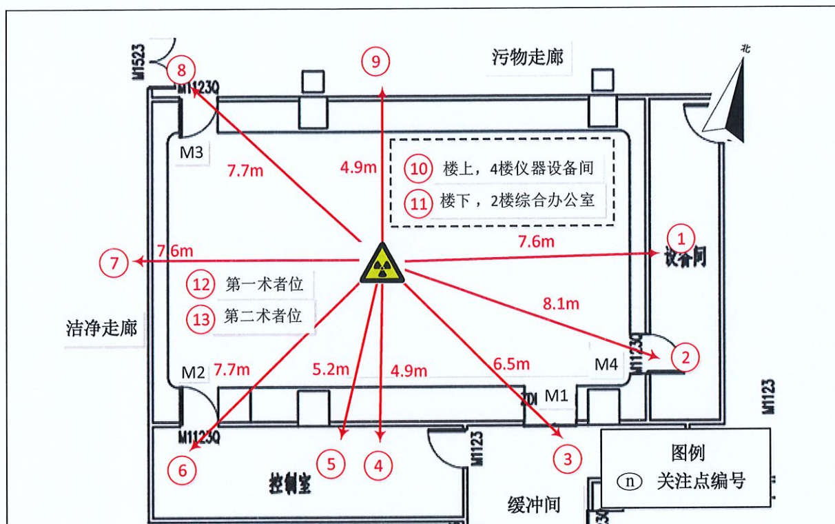
图 11-1 本项目 DSA 计算点位示意图
