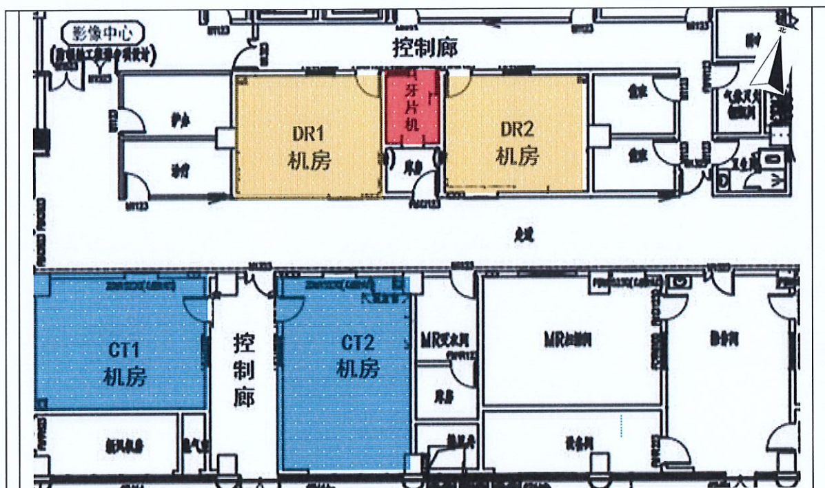
图 10-3 本项目 1 楼辐射工作场所（CT、DR、牙片机）平面布置图
