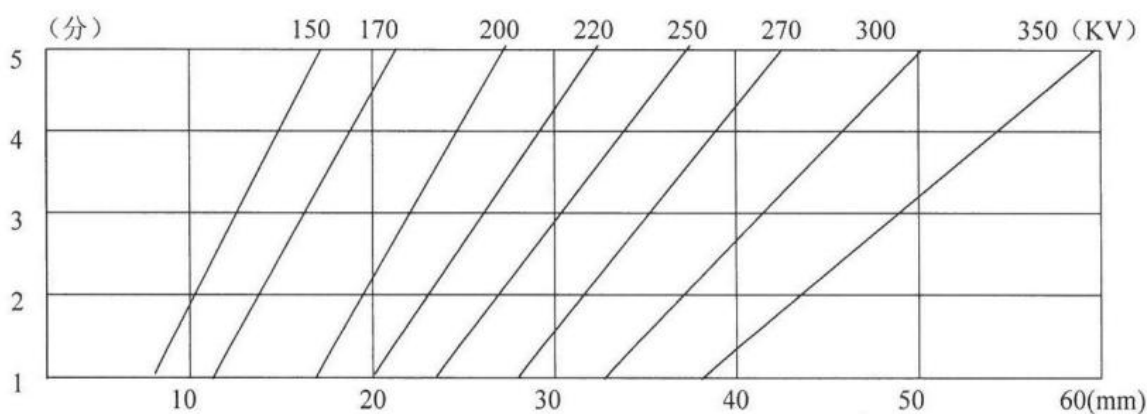
图 9-5 定向 X 射线探伤机曝光曲线图
