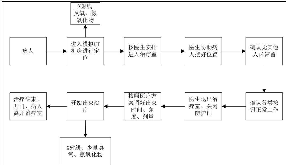
图 9-3 医用直线加速器放疗工作流程及产污环节示意图
