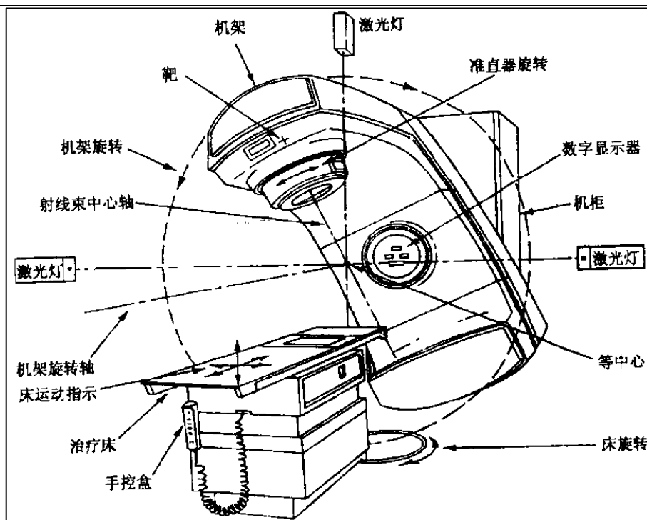
图 9-2 医用直线加速器基本结构示意图
