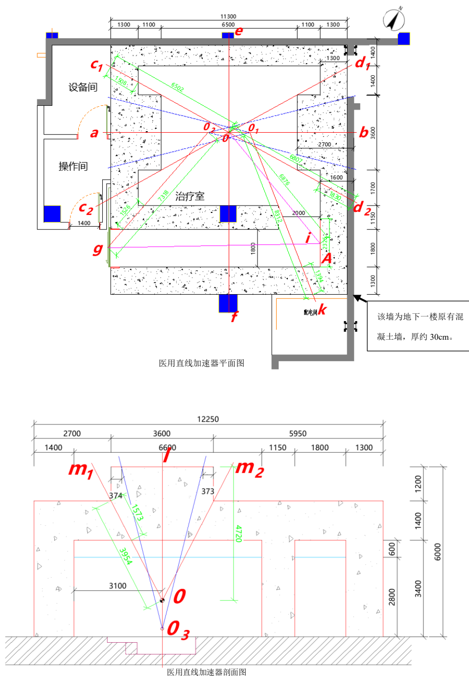
图 11-1 医用直线加速器机房估算点位示意图
