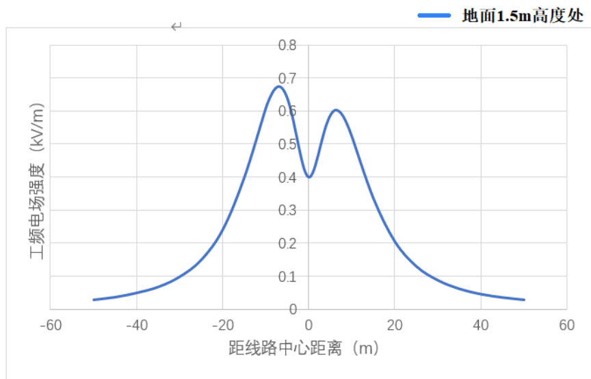
图 3.1-5 本期 110kV 架空线路工频电场强度变化趋势图
