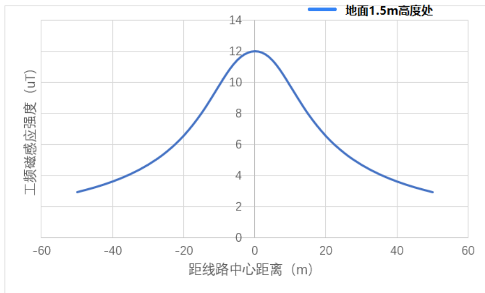
图 3.1-6 本期 110kV 架空线路工频磁感应强度变化趋势图
