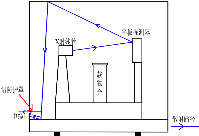
图 11-4 本项目工业 CT 装置电缆口散射示意图
