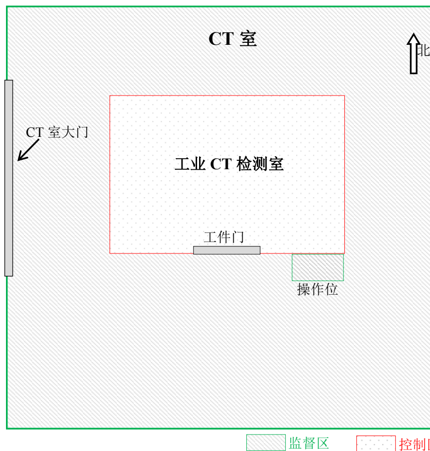
图 10-1 本项目 1 号 X-eye 7000BN 型工业 CT 装置监督区及控制区示意图
