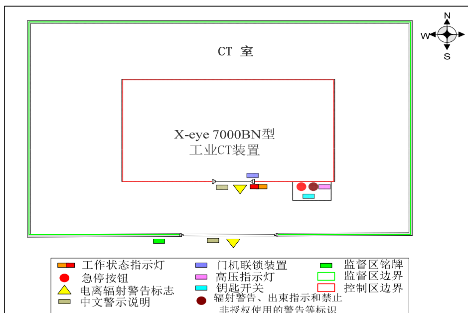
图 10-3 辐射安全设施平面布置示意图
