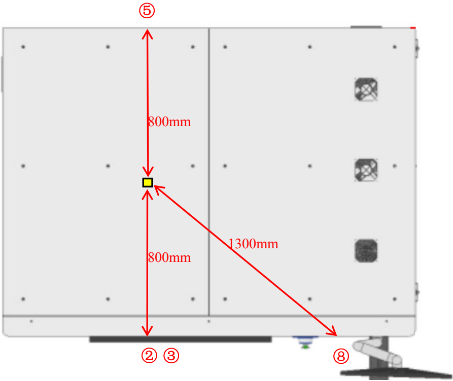
图 11-1 X-eye 7000BN 型工业 CT 装置关注点位示意图（2）
