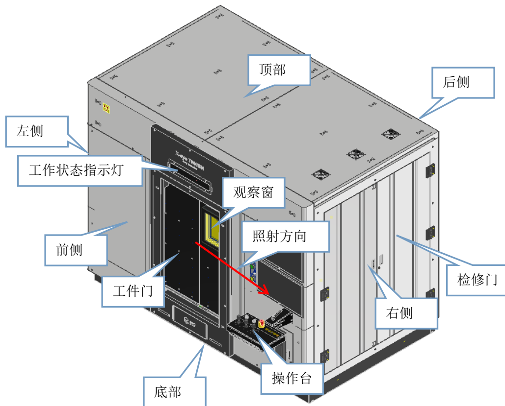
图 9-1 本项目 X-eye 7000BN 型工业 CT 装置样式图 (2)
