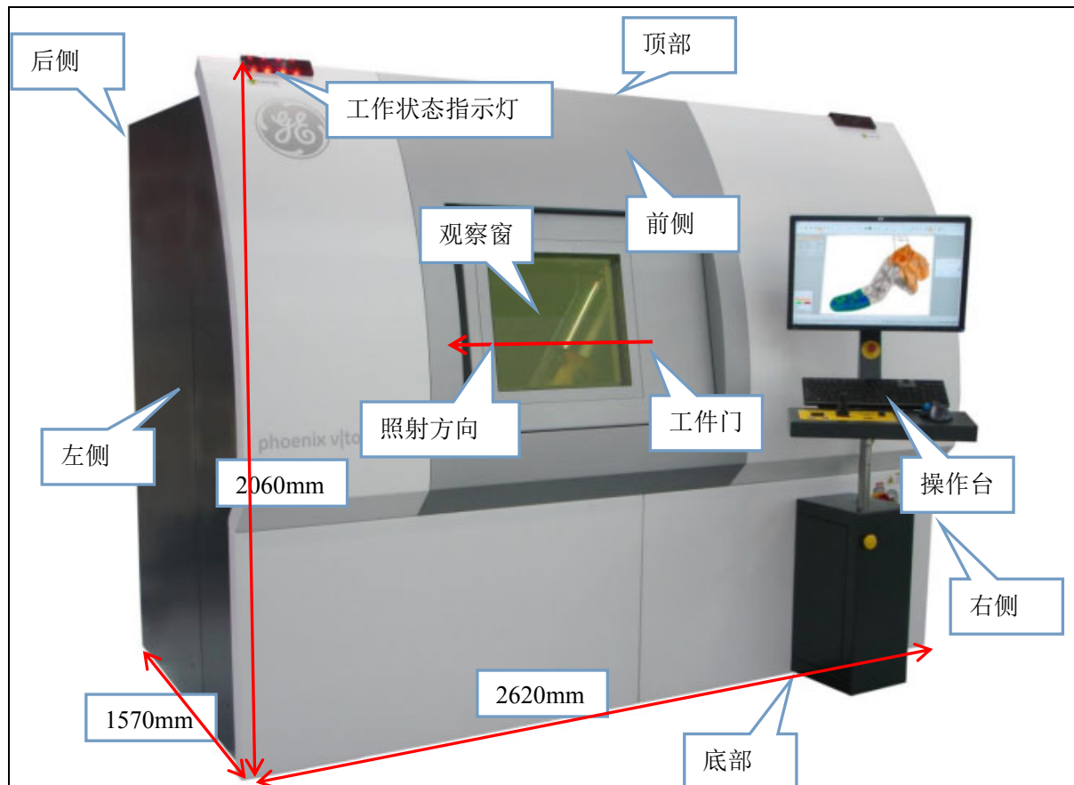
图 9-1 本项目 v|tome|x m 300/180 型工业 CT 装置样式图
