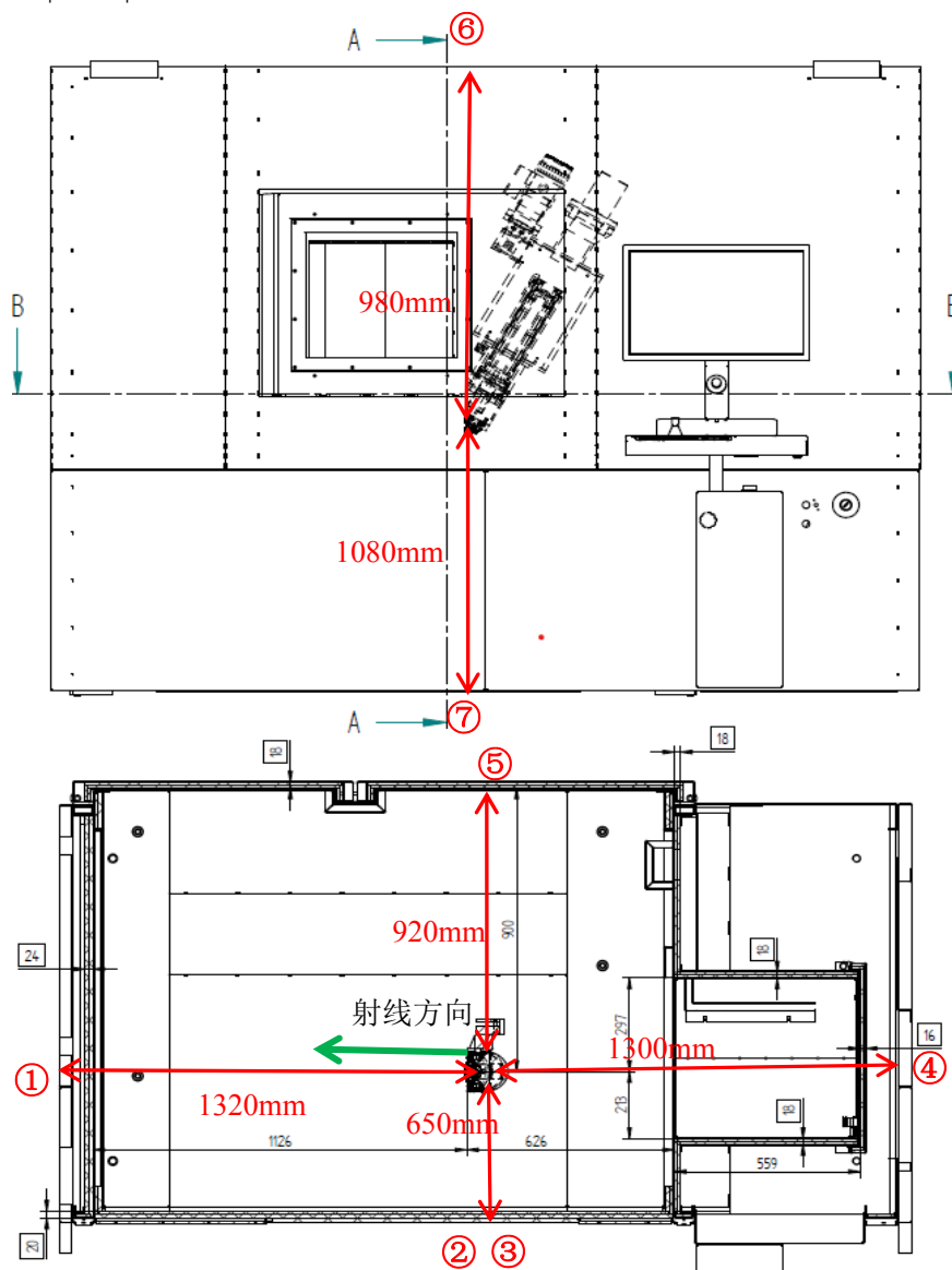
图 11-1 v | tome | x m300/180 型工业 CT 装置关注点位示意图
