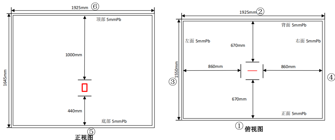
图 11-2 VT-X750 型工业 CT 检测装置辐射防护计算参考点为示意图
