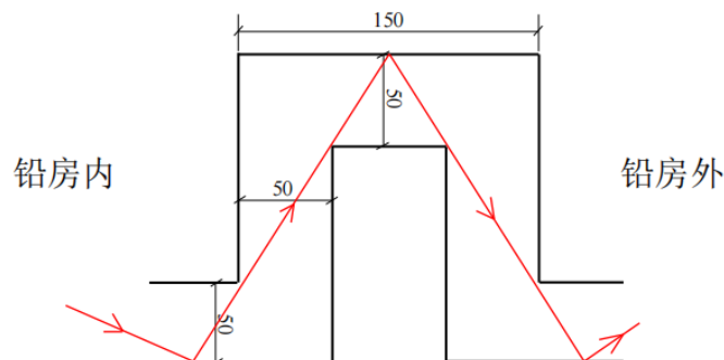
图 11-3 工业 CT 检测装置穿墙线管散射路径
