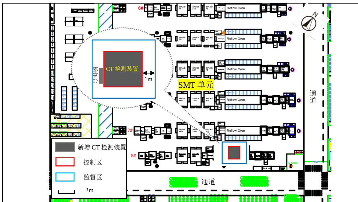
图 10-1 本项目 EF 电子车间 SMT 单元平面布局及分区示意图
