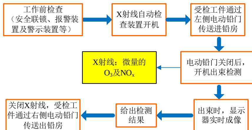
图 9-3 工业 CT 检测装置工作流程及产污环节示意图
