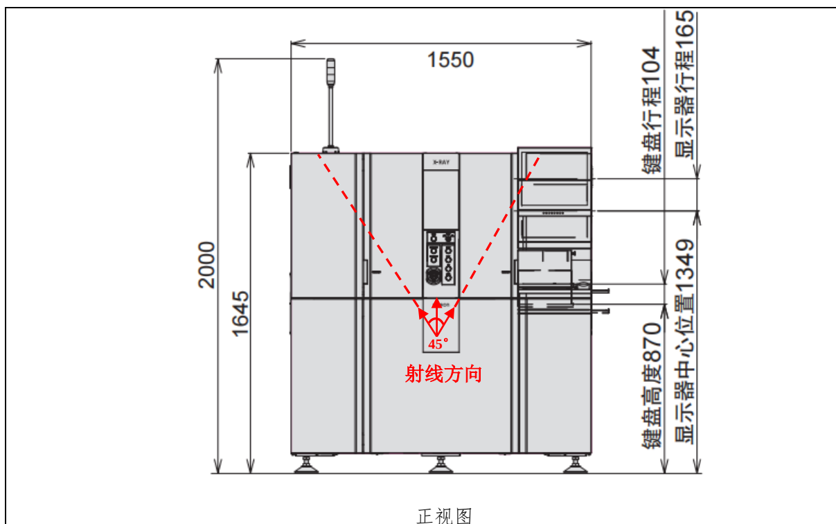
图 11-1 VT-X750 型工业 CT 检测装置设计示意图
