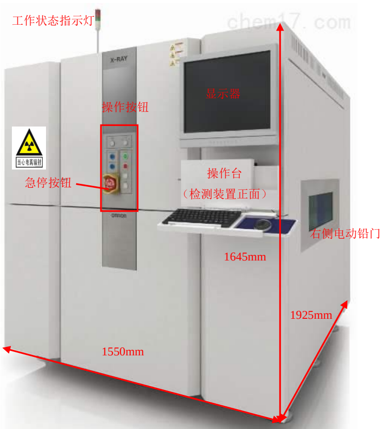
图 9-1 本项 VT-X750 型工业 CT 检测装置外观图
