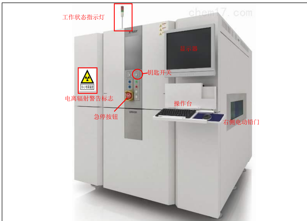
图 10-2 本项目辐射安全设施布设示意图
