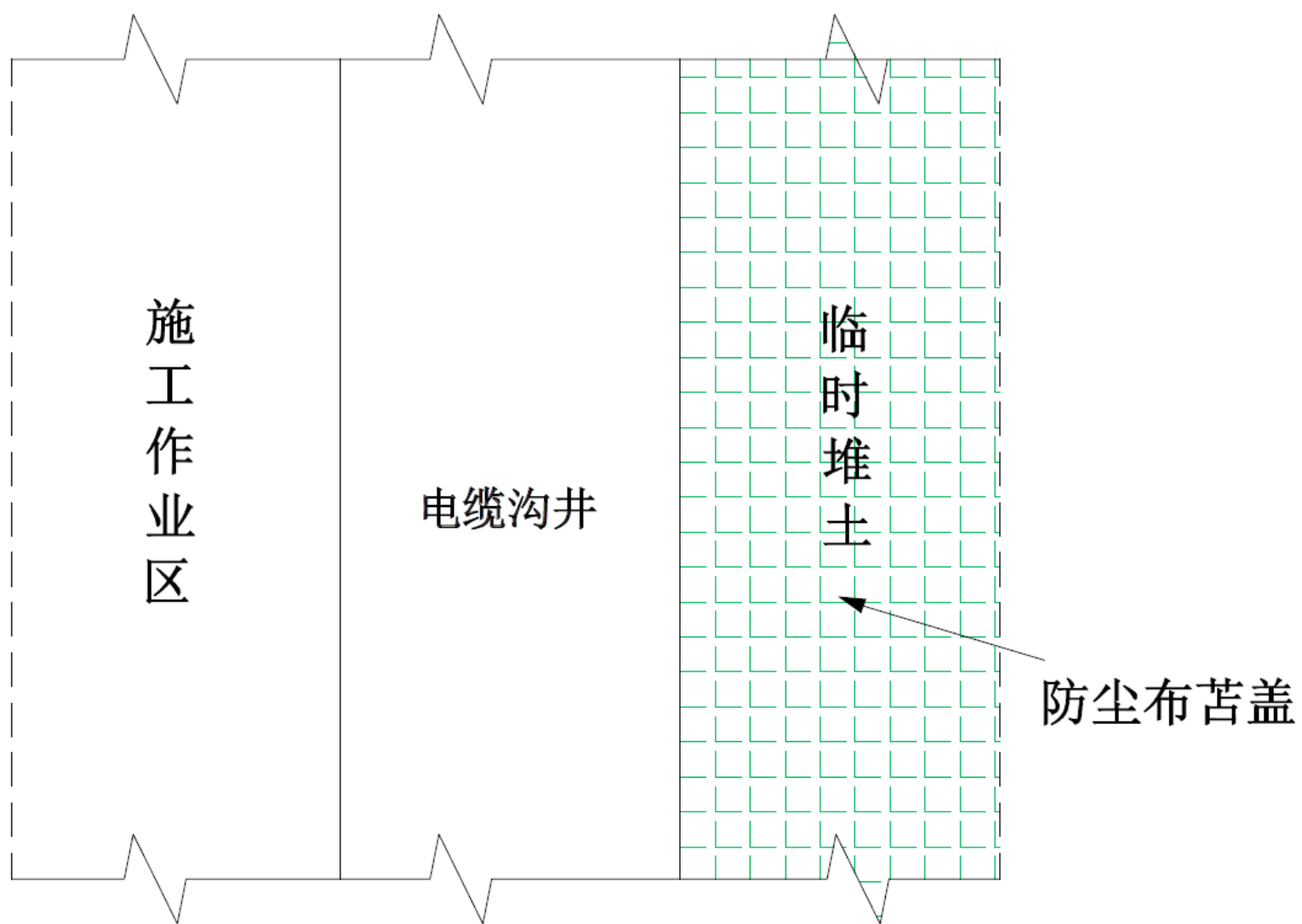
附图8 生态环境保护典型措施设计示意图（2）（堆土苫盖）
