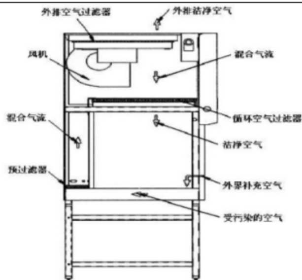
图 4-1 生物安全柜工作原理示意图
