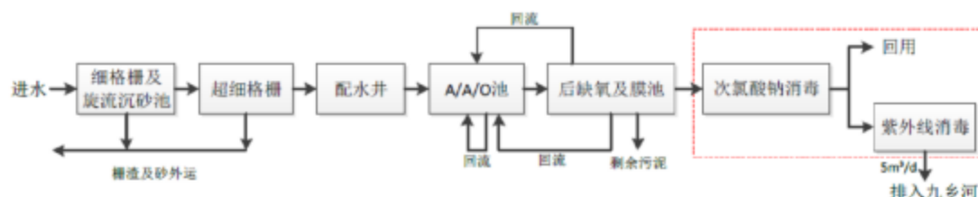
图 4-3 仙林污水处理厂工艺流程图
