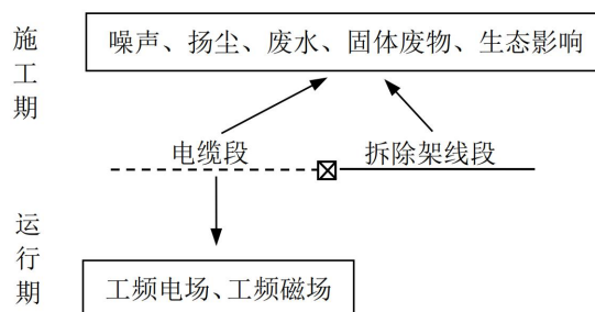
图2-1 本项目工艺流程及产污环节图
