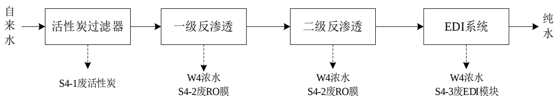
图 2-6 纯水制备生产工艺流程图
