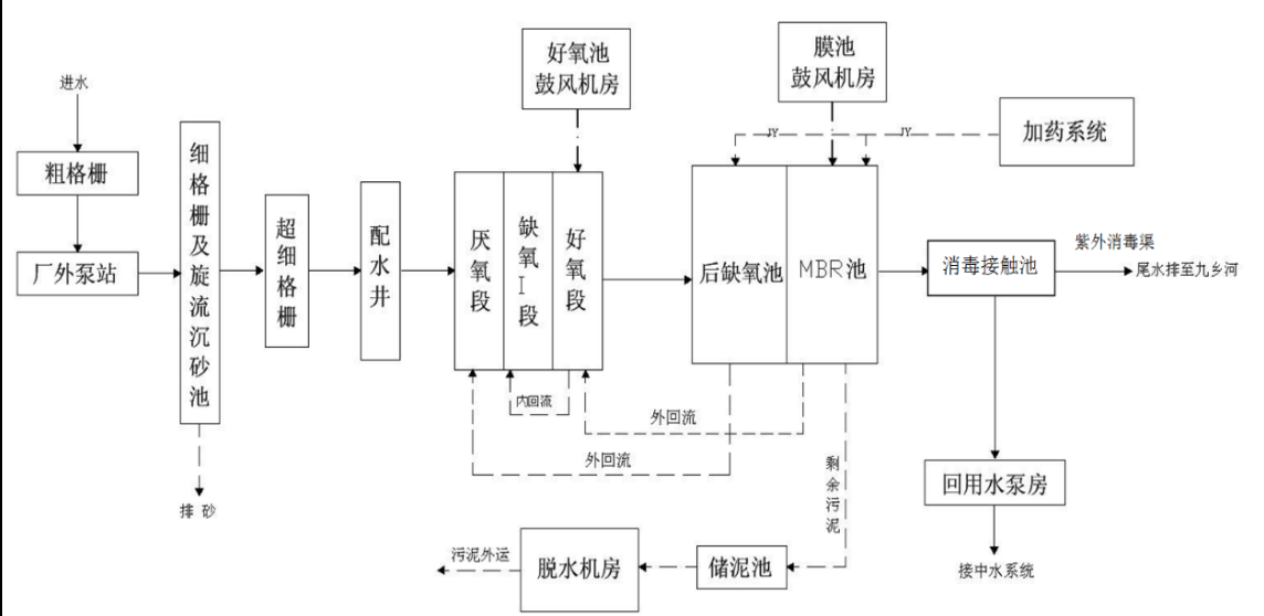
图 4-2 仙林污水处理厂工艺流程图
