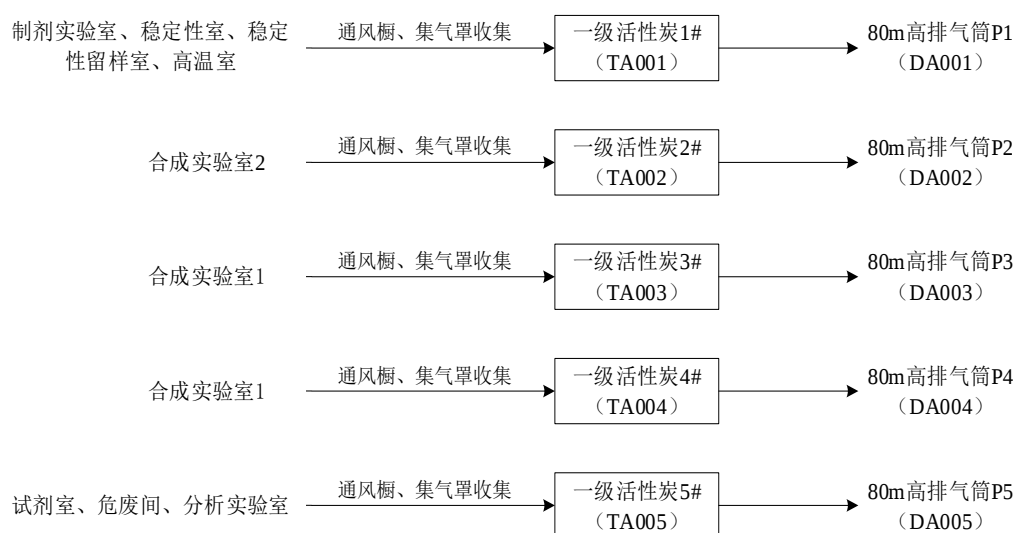
图 6-1 废气收集处理流程图
