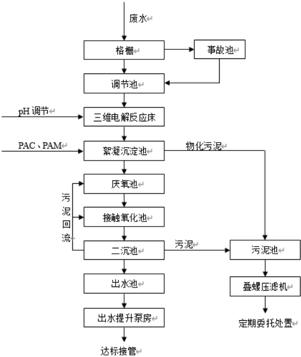
图 4-1 园区污水处理站工艺流程图
