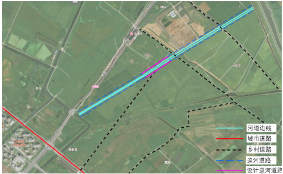
图 2-5 设计巡查道路图
