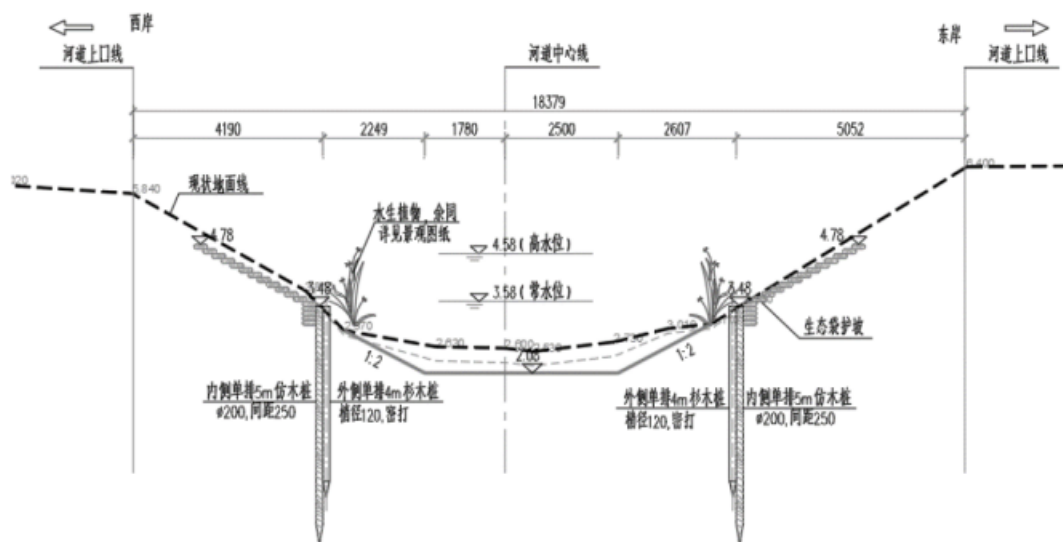
图 2-9 现状河段梯形断面
