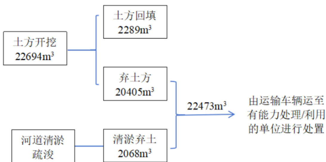
图 2-1 土方平衡图
