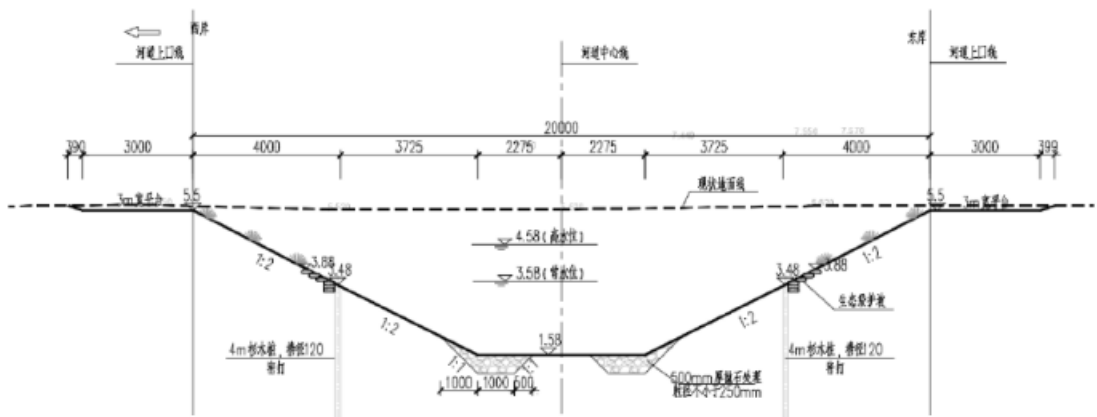
图 2-4 新开挖河段梯形断面
