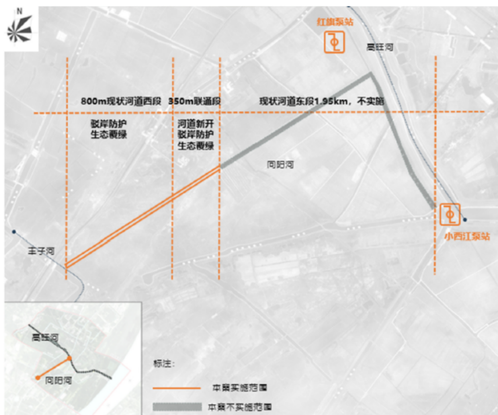
图 2-3 向阳河生态保护修复平面图
