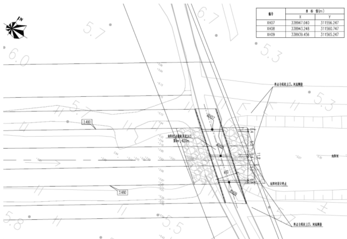
图 2-7 箱涵平面布置图 (3#)
