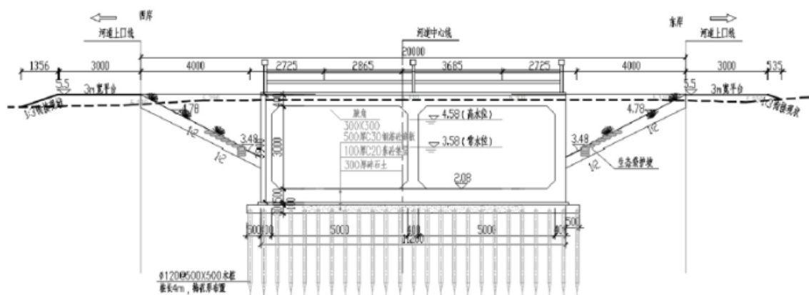
图 2-8 箱涵断面图
