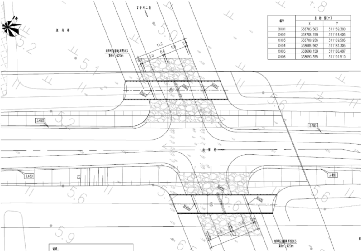
图 2-6 箱涵平面布置图（1#、2#）
