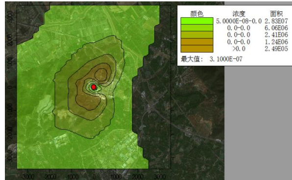
图 6.1.3-14 Hg 全时段浓度贡献值分布图 (mg/m 3 )
