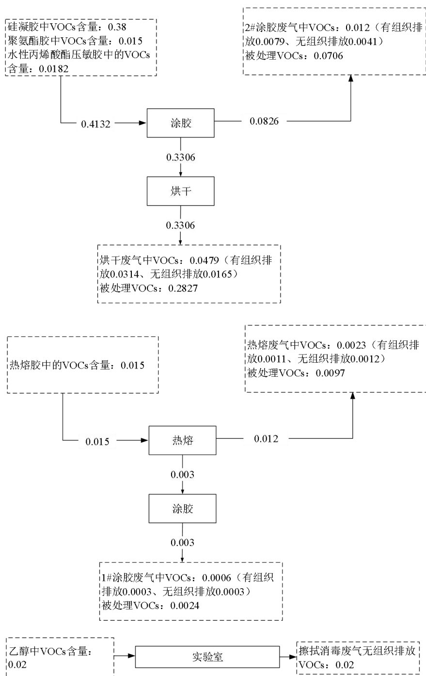
图 2-2 本项目 VOCs 平衡图 (单位: t/a)
