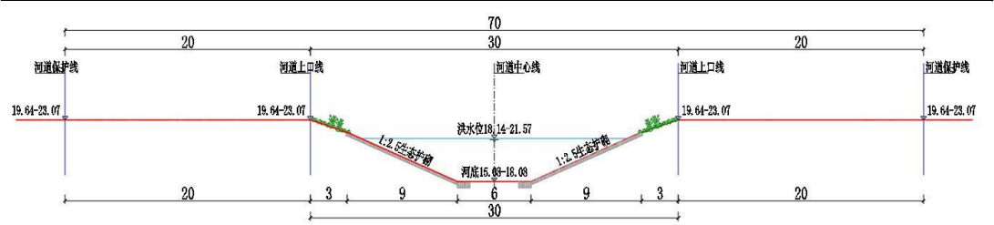
图 2-6 新建段河道典型设计断面
