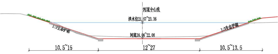
图 2-6 新建段河道典型设计断面
