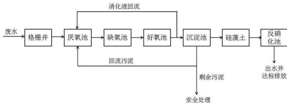
图 4-1 洪蓝污水处理厂工艺流程示意图
