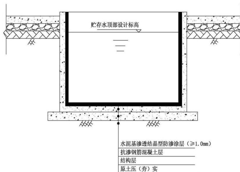
图 6.5.3-2 水池防渗结构示意图
