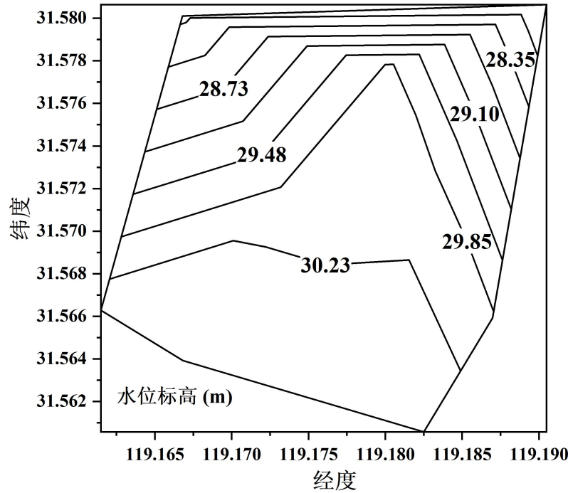
图 5.2.5-5 地下水等水位线图
