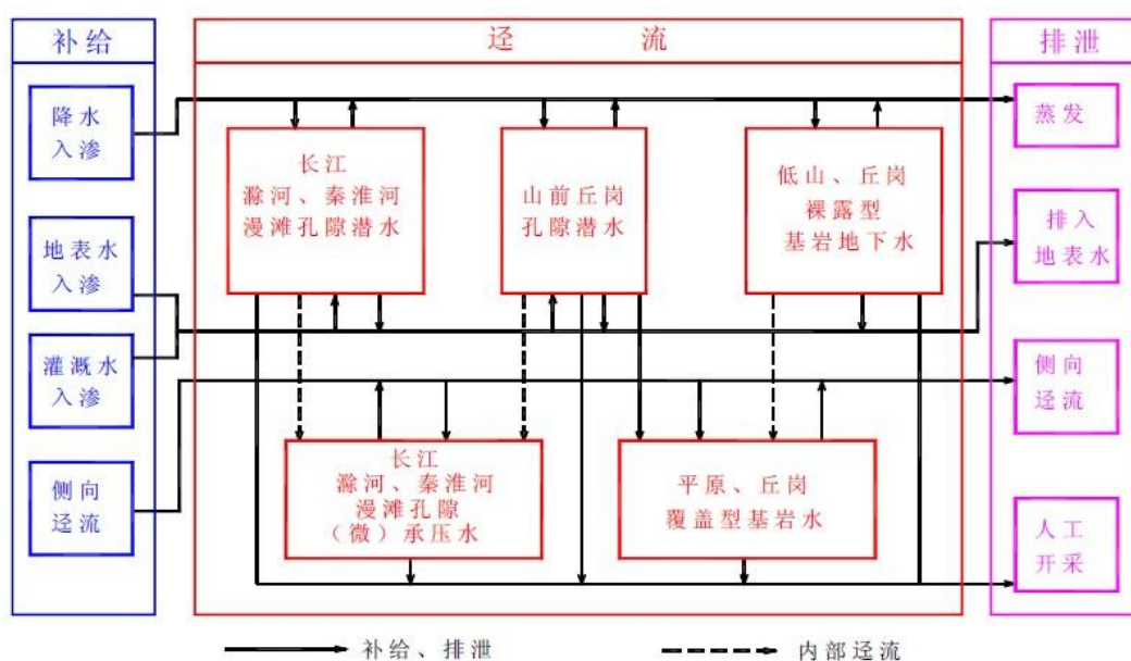
图 5.2.5-2 地下水补给、径流、排泄关系略图
