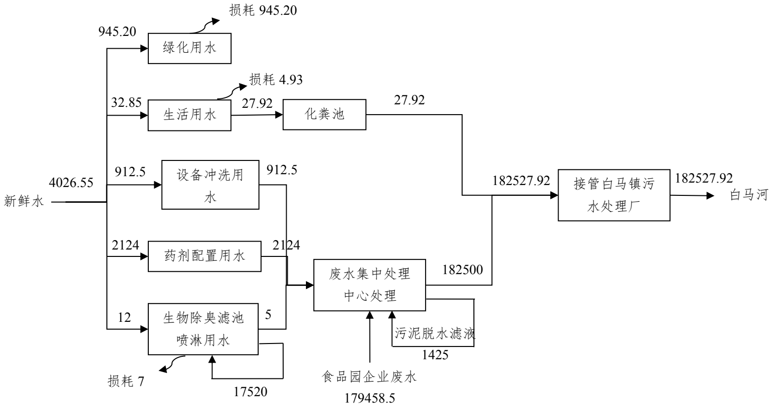
图 3.6.2-1 建设项目水平衡图（单位：t/a）
