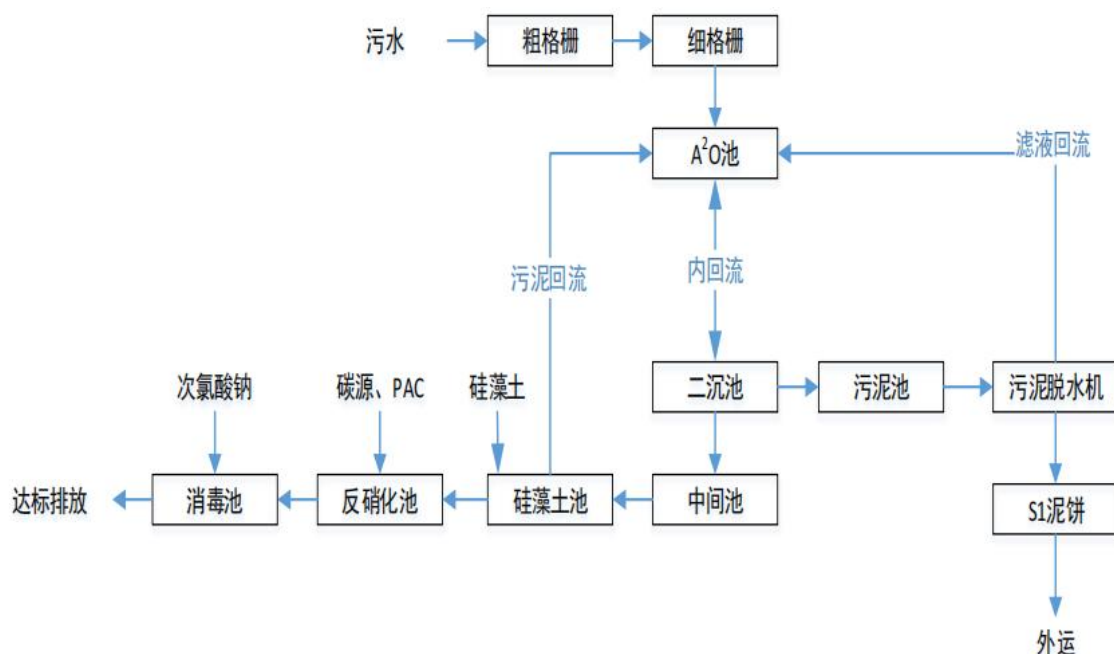
图 2.7.3-1 白马镇污水处理厂处理工艺流程图
