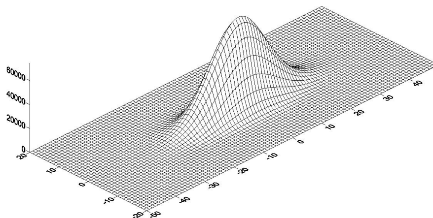
图 5.2.5-9 非正常工况下 20 年后 \text{COD}_{\text{Mn}} 影响范围
