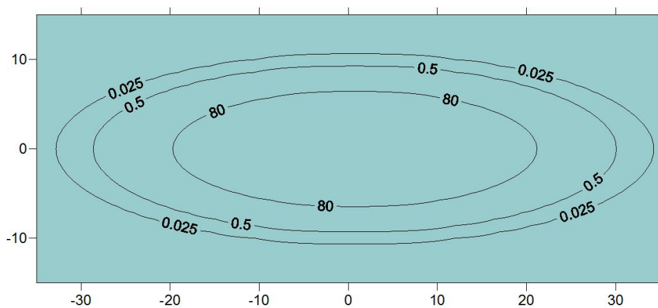
图 5.2.5-11 非正常工况下 1000d 后氮氮影响范围
