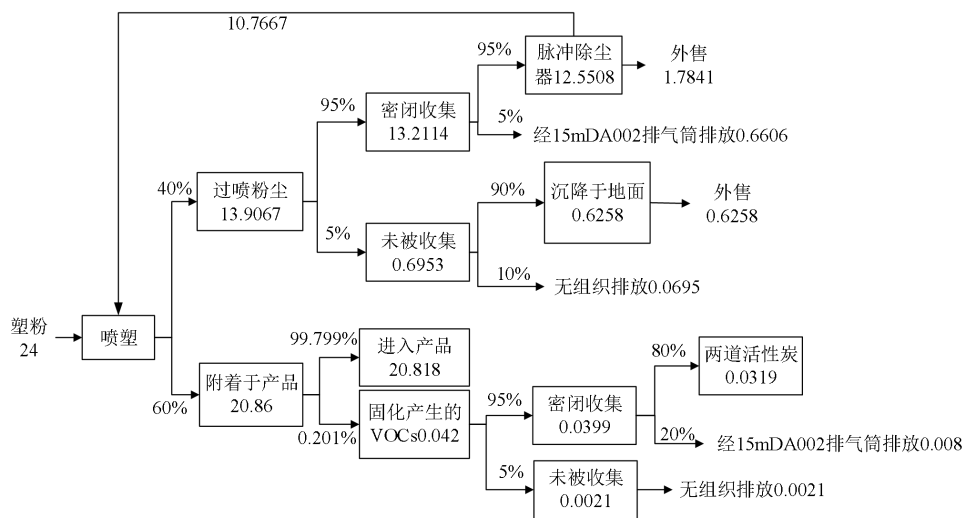
图 2-1 项目塑粉平衡图(单位: t/a)
