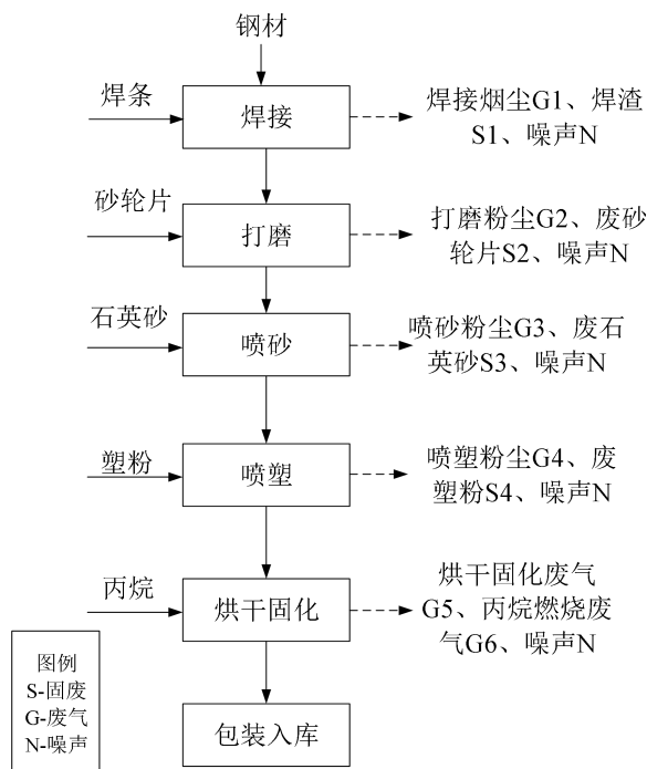
图 2-4 生产工艺流程图
