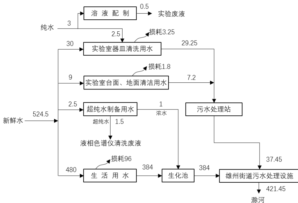
图 2-1 建设项目营运期水平衡图（单位：t/a）
