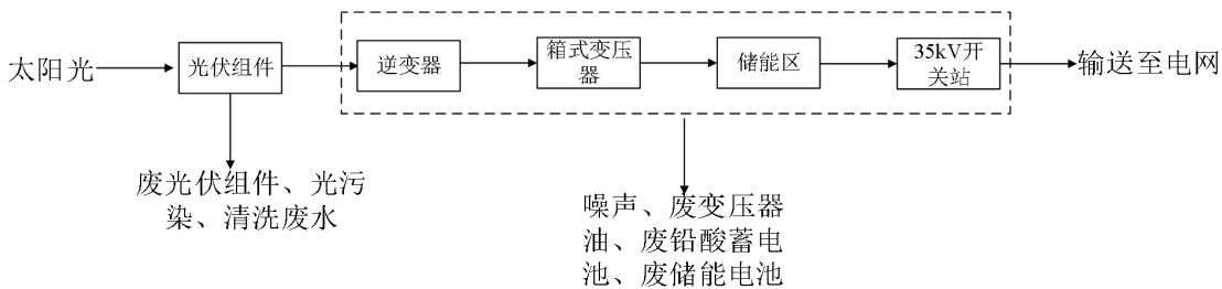
图 4-1 项目运营期工艺流程及产排污环节示意图
