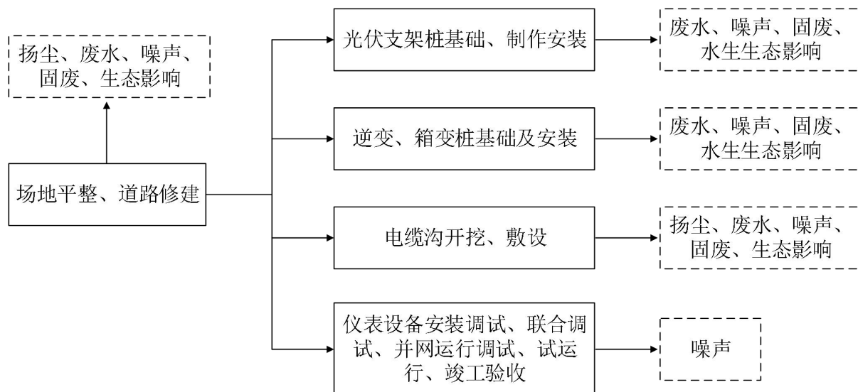
图 2-2 施工工艺流程及产污环节图
