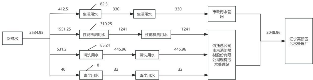
图 2-1 本项目给排水平衡图 (t/a)
