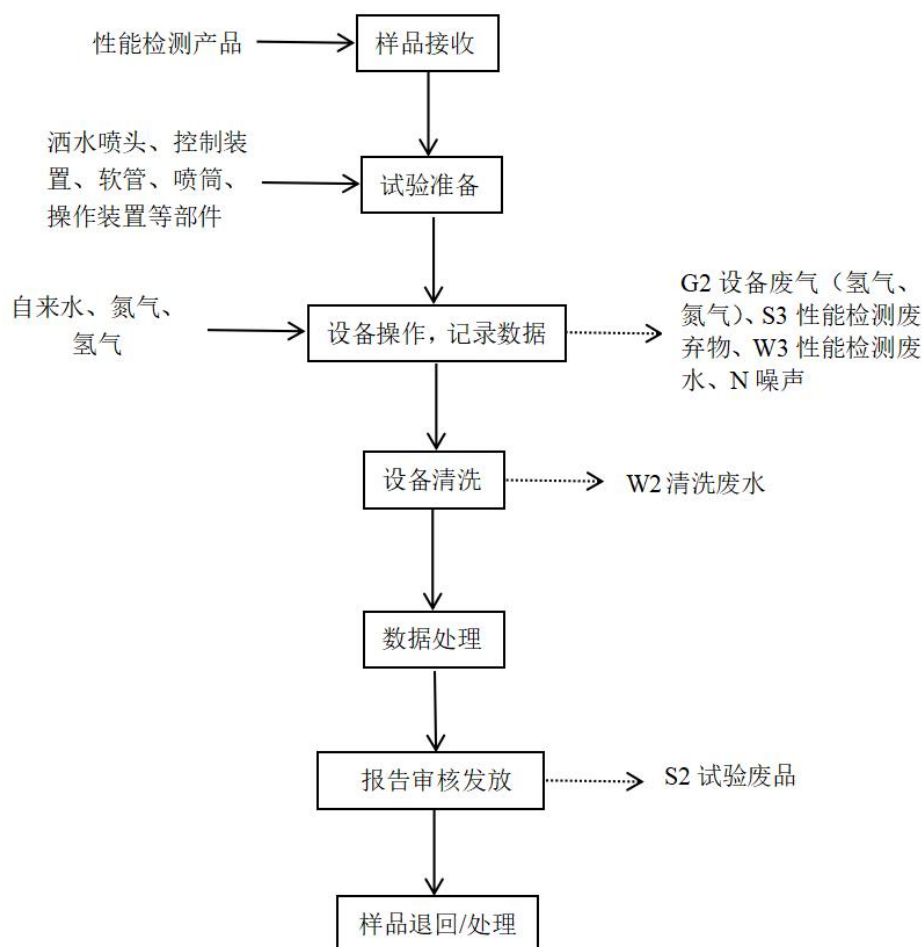
图 2-3 消防产品性能检测流程图及产污环节
