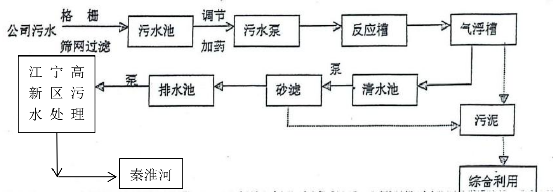
图 4-1 生产废水处理设施污水处理工艺流程图
