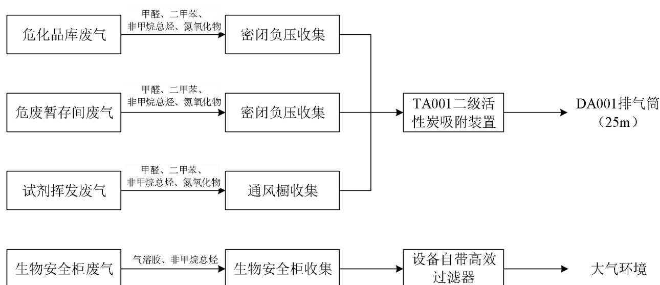
图2-1 本项目废气治理工艺流程图
