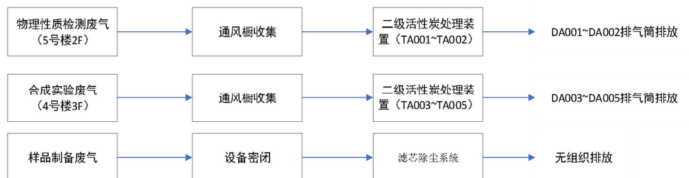
图 2-4 现有废气流程图
