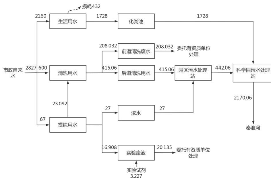
图 2-5 现有项目水平衡图 (t/a)
