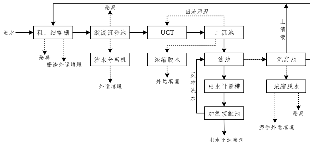
图 4 城东污水处理厂工艺流程图
