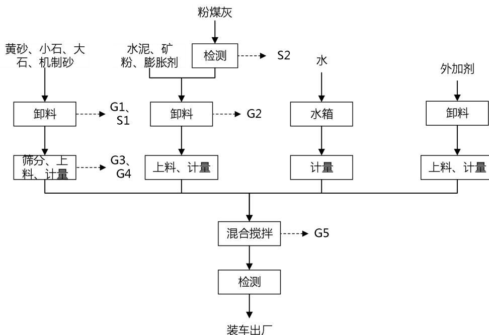
图 2-3 生产工艺流程及产污环节图
