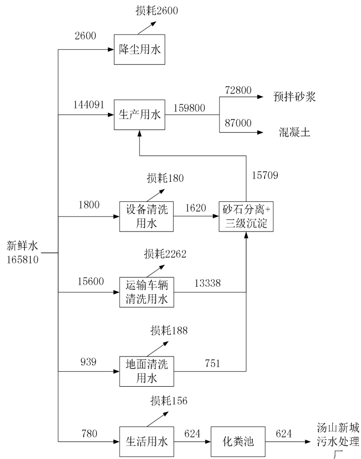
图 2-2 扩建后全厂水平衡图 (m³/a)
