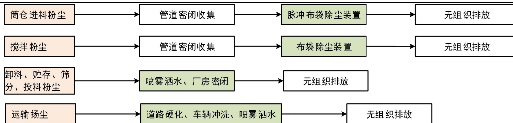
图 4-2 扩建项目废气处理工艺图
