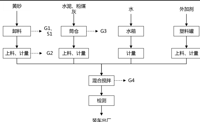
图 2-4 现有项目生产工艺流程及产污环节图
