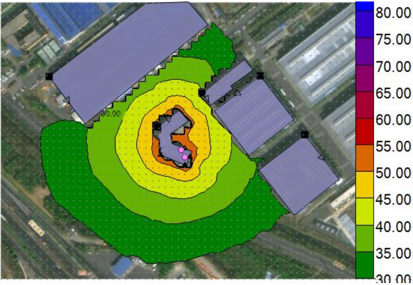
图 4-3 企业厂界噪声预测结果等值线图
