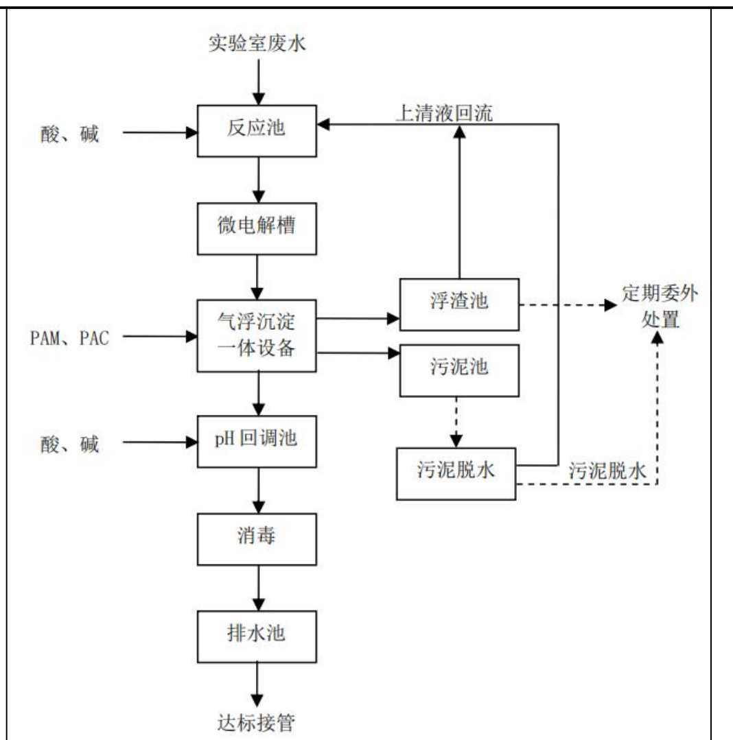
图 4-1 慧科园区污水处理站废水处理工艺流程图
