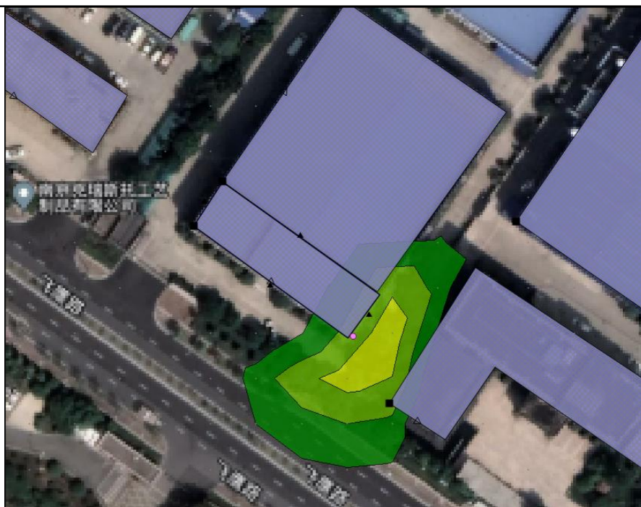
图 4-3 厂界噪声预测结果图
