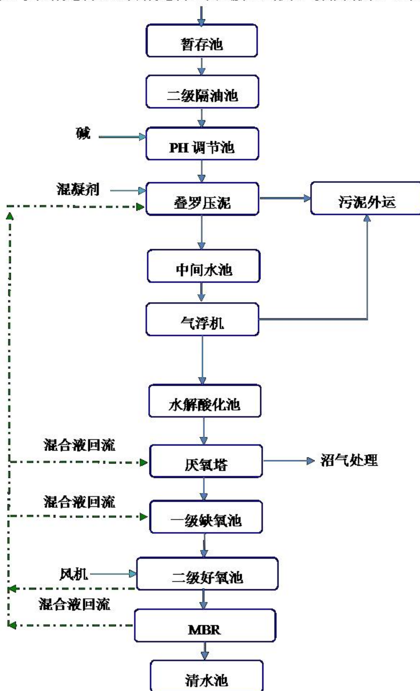
图 4-1 污水处理工艺流程图 t/a
