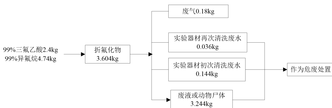
图 2-5 氟化物物料平衡图（单位：kg/a）
