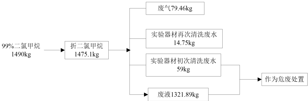
图 2-2 二氯甲烷物料平衡图（单位：kg/a）
