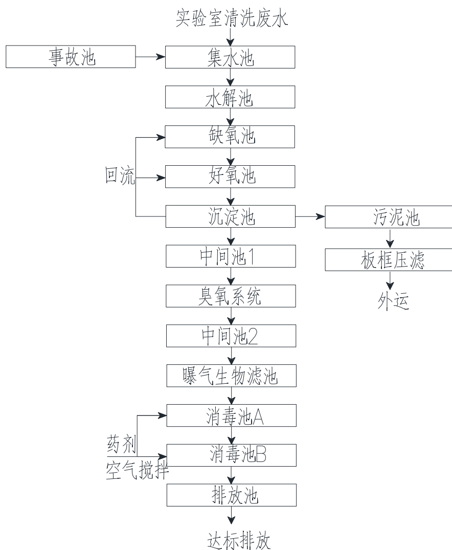
图 4-1 天印健康创新园污水处理站工艺流程图
