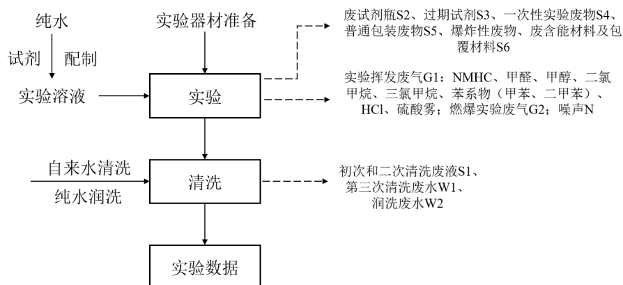
图 2-5 化学实验流程及产污环节图
