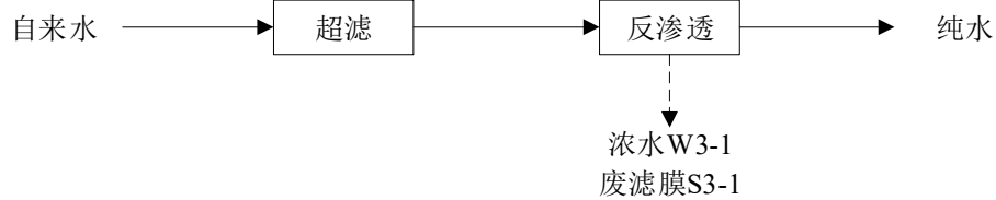
图2-4纯水制备工艺流程图
