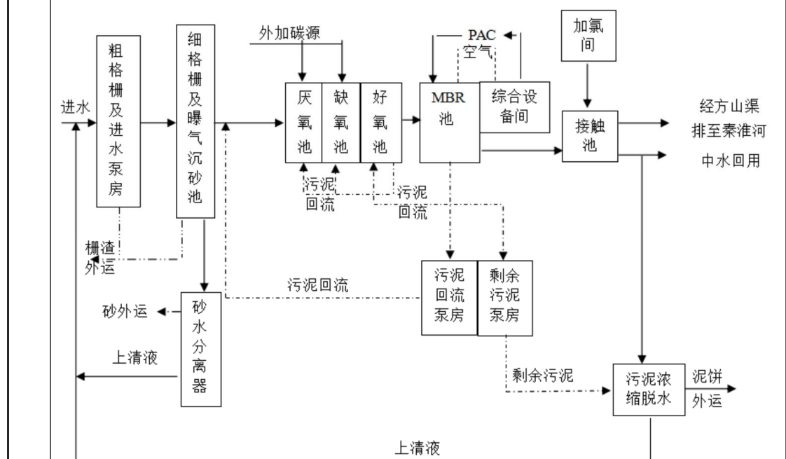
图4-2科学园污水处理厂三四期工程工艺流程图
