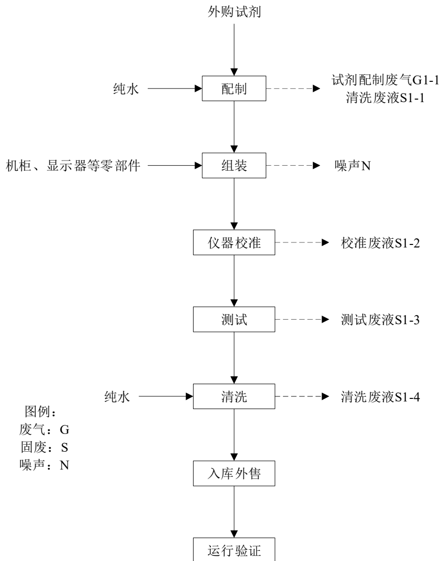
图2-2本项目环境自动在线监控仪器生产工艺流程图
