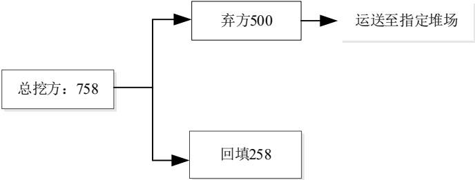
图 4-1 本项目土石方平衡图 单位：m³
