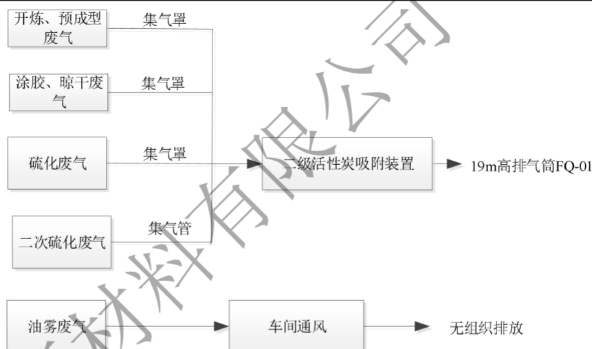
图 4-1 本项目废气收集处理工艺图
