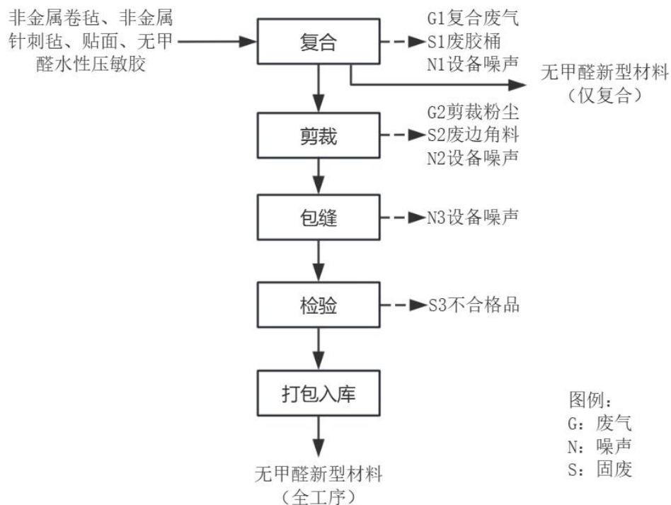
图 2-2 无甲醛新型材料生产工艺流程图及产污环节
