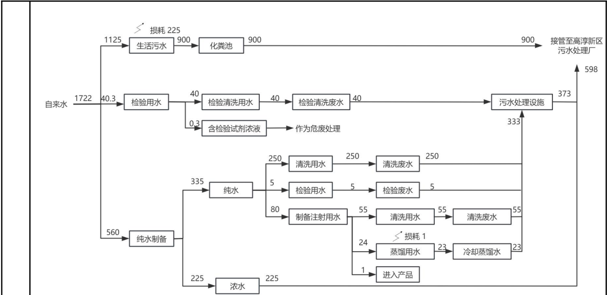
图 2-1 建设项目用水平衡图 (t/a)
