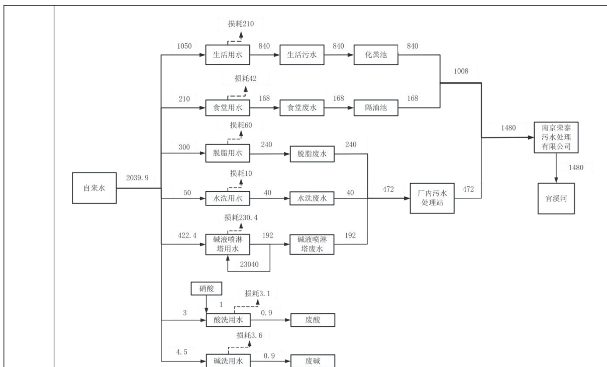
图 2-5 现有项目水平衡图 单位: t/a
