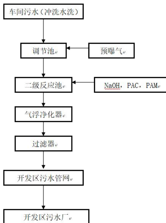
图 4-1 污水处理站处理工艺
