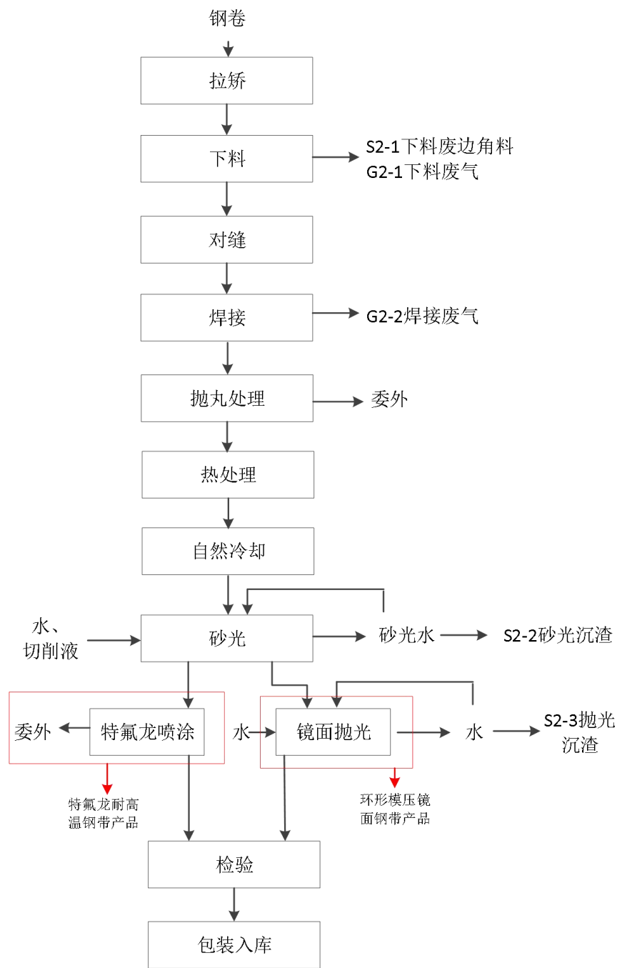
图 2-3 环形模压钢带生产线工艺流程图 环形模压钢带生产线工艺流程说明
