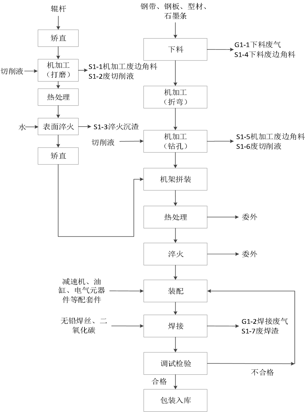
图 2-2 双钢带连续压机生产线工艺流程图 双钢带连续压机生产线工艺流程说明
